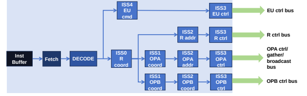
Figure 17: TIU Pipeline.
